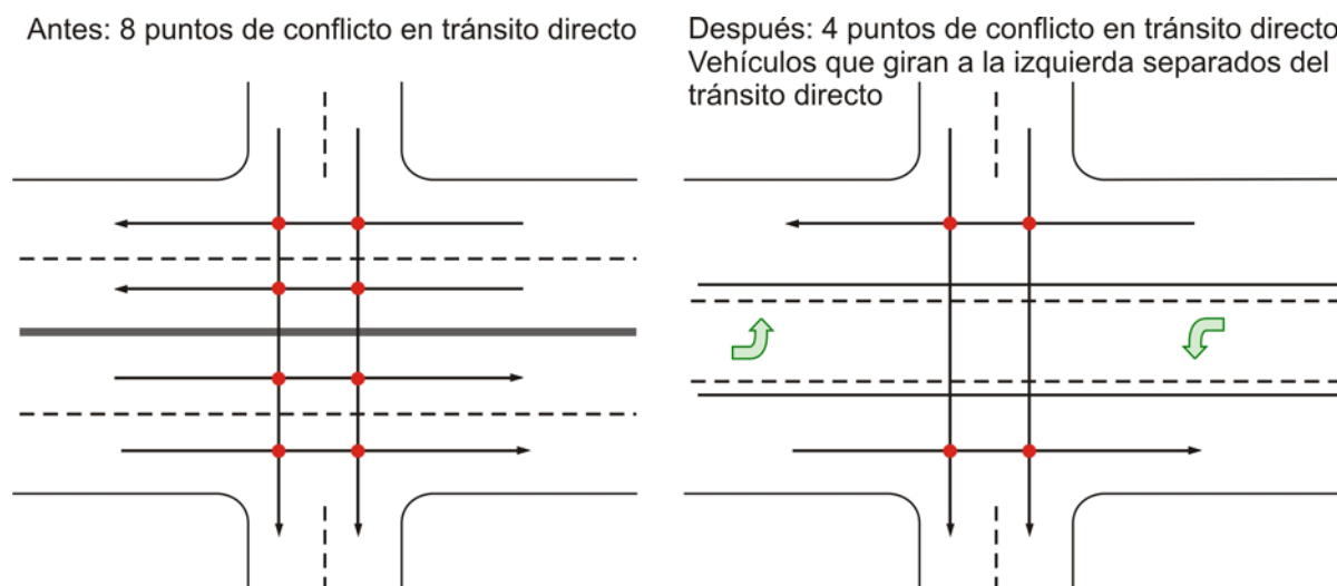
Figura 2.41 Reducción de puntos de conflicto en tránsito directo por la conversión de una calzada indivisa de cuatro carriles a una sección transversal de tres carriles.
