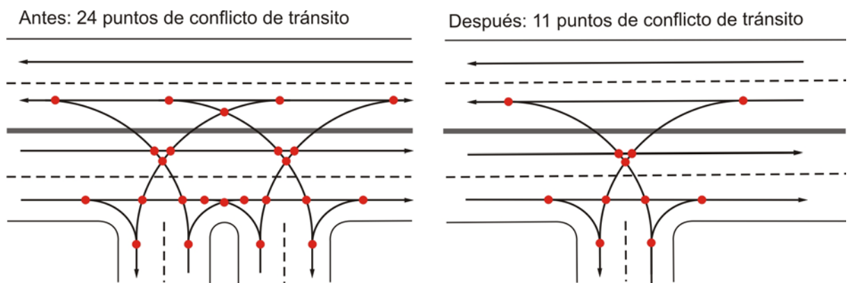
Figura 2.40 Reducción de puntos de conflicto por la consolidación de accesos de dos accesos cercanamente espaciados en una calzada indivisa de cuatro carriles.
